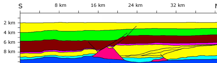
(d) Present Day
