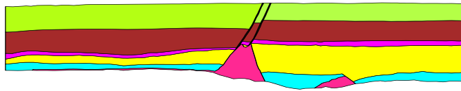
(d) Messinian (6 Ma)
